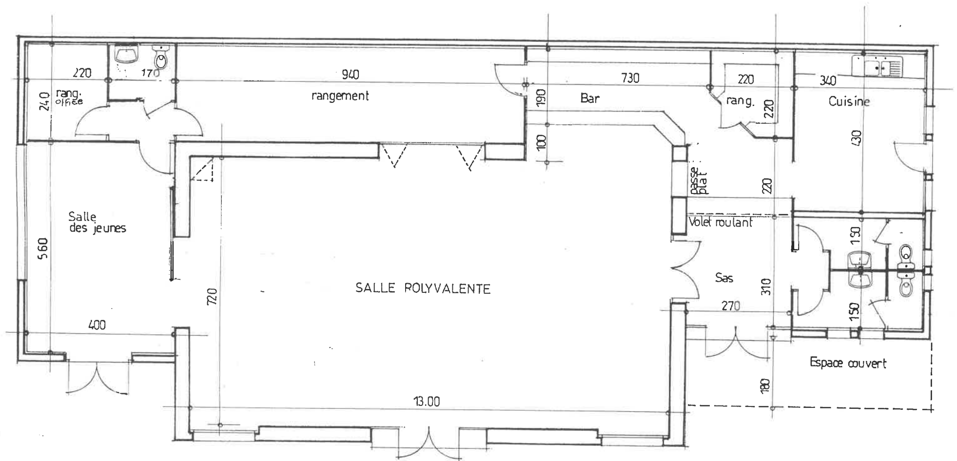
Plan de salle polyvalente et annexes
